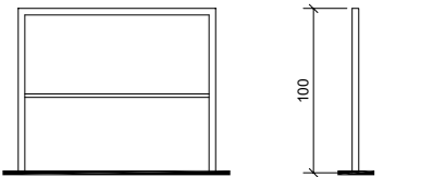
DETALL BARANA METÀL·LICA E: 1/50 cotes en cm
