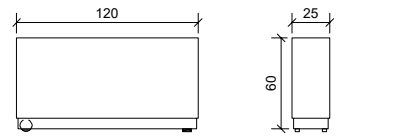
DETALL JARDINERA GIRONA E: 1/50 cotes en cm
