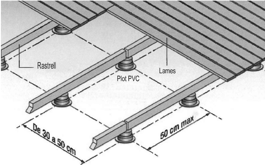
DETALL ORIENTATIU DE L'ESTRUCTURA SOBRE PLOTS
